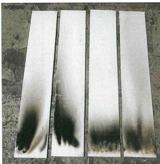
Рис.1 – Образцы после испытаний
